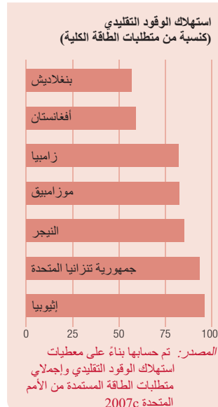
الشكل 1.8 الاعتماد على وقود الكتلة الأحيائية في العديد من الدول
