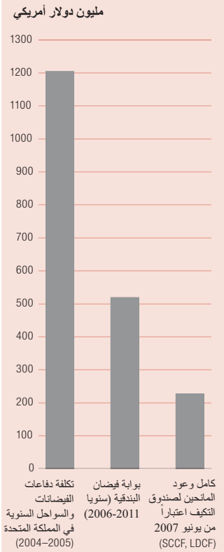
الشكل 4.5 أفوق استثمارات الدول المتطورة صندوق التكيف الدولي
