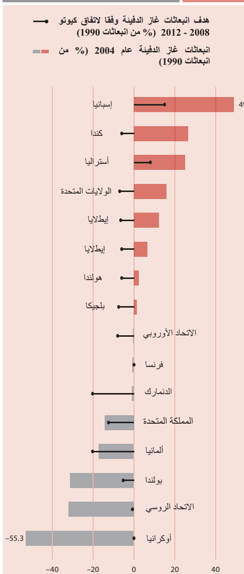
الشكل 1.14 بعض الدول المتقدمة بعيدة كل البعد عن تحقيق أهداف التزامات كيوتو
